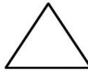
triângulo equilátero
